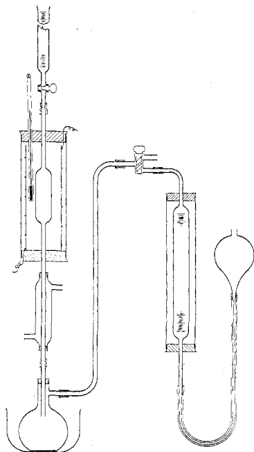
Fig. 1.—Apparatus.
